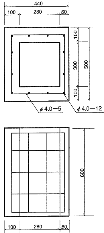
L型250BG、L型300G、特L型275G用 (旧タイプ)
