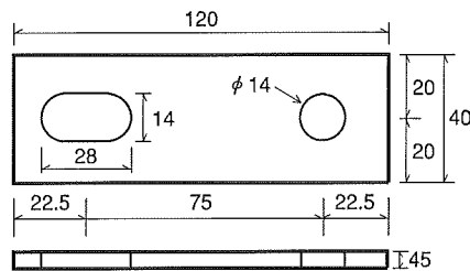
連結プレート詳細図
