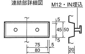
連結部詳細図
