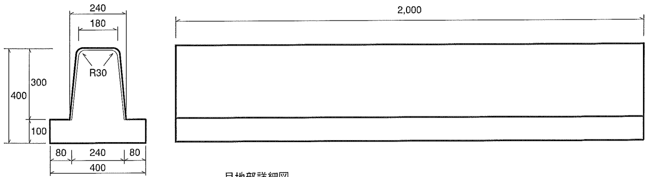
目地部詳細図
